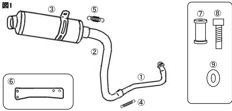
パーツリスト(梱包内容)
