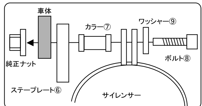
模式図の為、実際のボルト・ナットと形状が異なります
